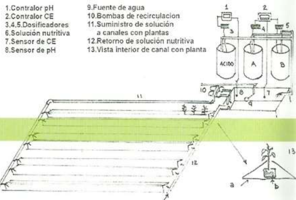
Figura 14. Técnica de la película nutritiva (NFT)
